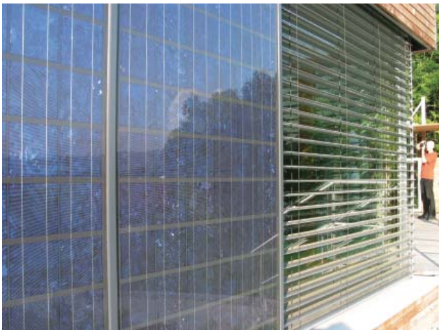
Obr. 3 Větší okna pasivního domu jsou zpravidla doplněna venkovním stíněním. V této variantě jsou do fasády zabudovány také fotovoltaické panely.
