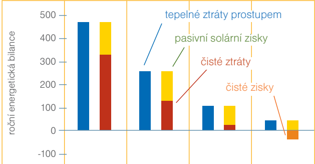
Obr. 6 Porovnání různých druhů zasklení z hlediska celkové roční energetické bilance. Jak je vidět, sebelepší izolační dvojskla jsou v konečném součtu ztrátová. Až použitím trojskel lze dosáhnout v pasivních domech stavu, kdy okna v otopné sezóně produkují zisky. Výše uvedené samozřejmě platí pro správnou orientaci hlavní prosklené plochy na jih. (Zdroj Passivhaus Institut)
