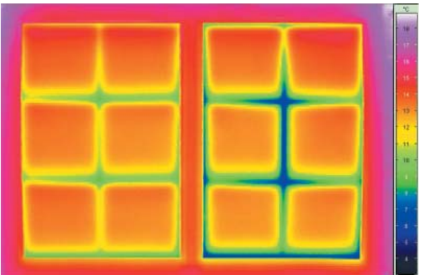
Obr. 8 Nepříjemné orosení okna na interiérové straně může být způsobeno více faktory, nejčastější je nízká povrchová teplota zasklení. Kvalitní okna a zasklení pro pasivní domy těmito problémy netrpí. Porovnání skel s teplým rámečkem (vlevo) a s běžným hliníkovým rámečkem (vpravo). (archív SGG Swisspacer)
