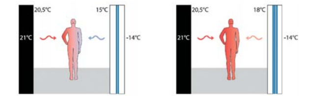
Obr. 4 Při použití prosklených ploch s nekvalitním zasklením je povrchová teplota okna nízká a v blízkosti okna je cítit nepříjemný chlad. Naopak při použití oken s parametry zasklení na úrovni pasivního domu je zajištěna tepelná pohoda.
